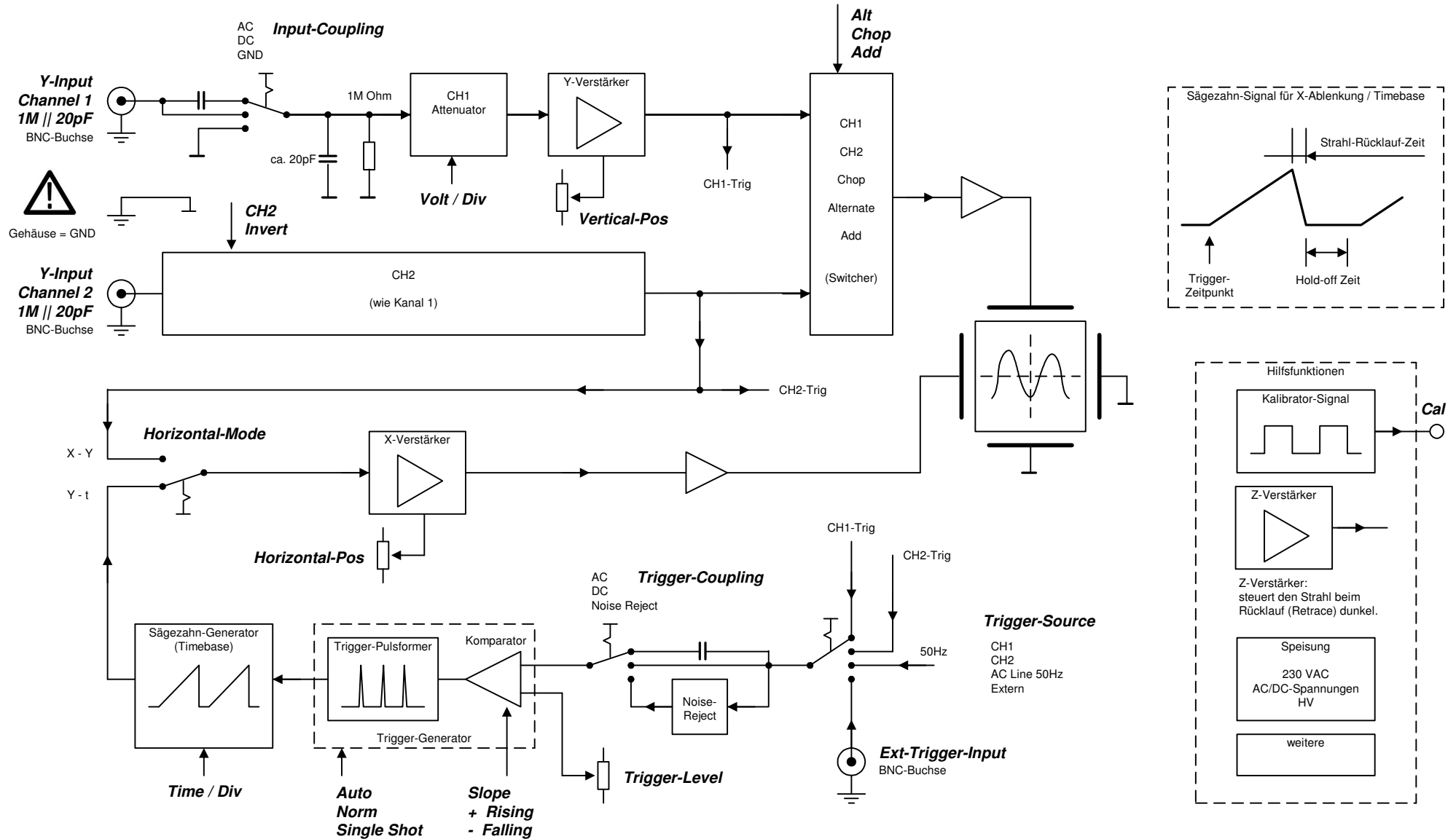
Vereinfachtes Blockdiagramm eines Analog-KOs (Tektronix-Bedienung)
