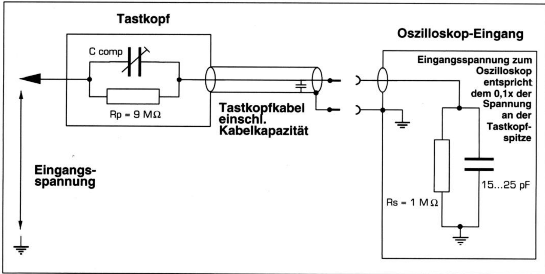
Abb. 43 Schaltbild für 10:1-Tastkopf
