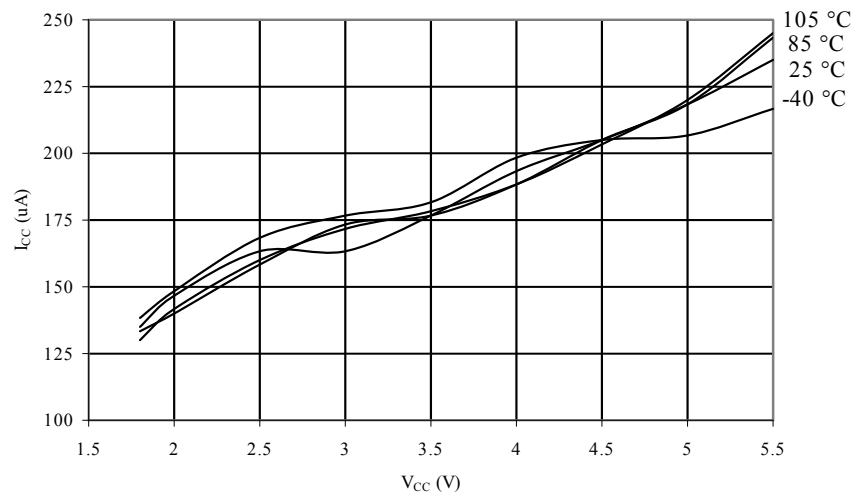
Figure 30-41. ADC Current vs. V CC (AREF = AV CC )
